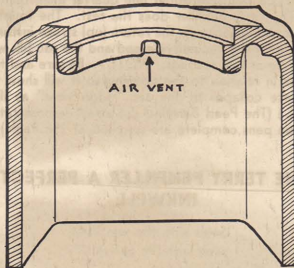
MODERNE PLASKON CASE
